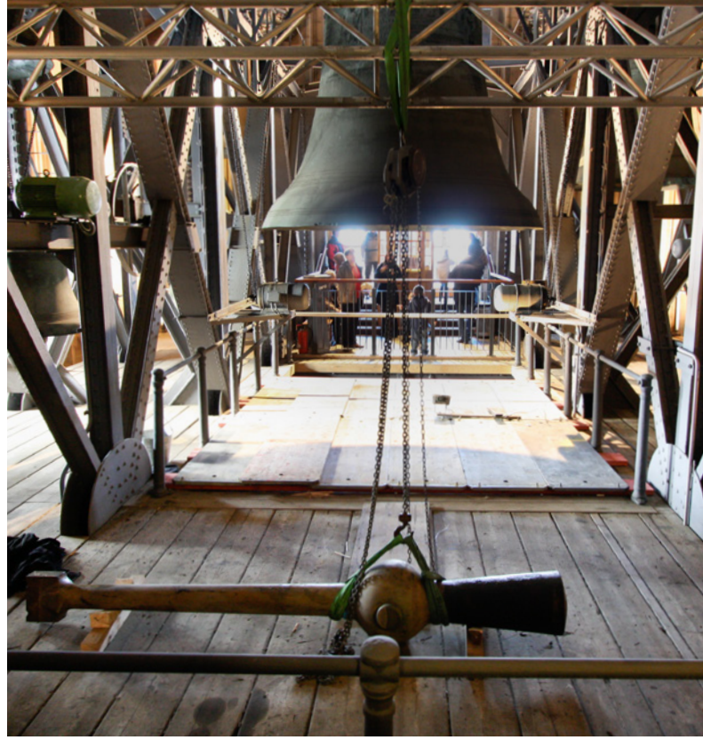
Petersglocke mit ausgebautem Klöppel: Die Petersglocke wurde 1923 von Heinrich Ulrich in Apolda als seinerzeit größte freischwingende Kirchenglocke der Welt gegossen und ersetzt seit 1924 die im ersten Weltkrieg eingeschmolzene Kaiserglocke.
